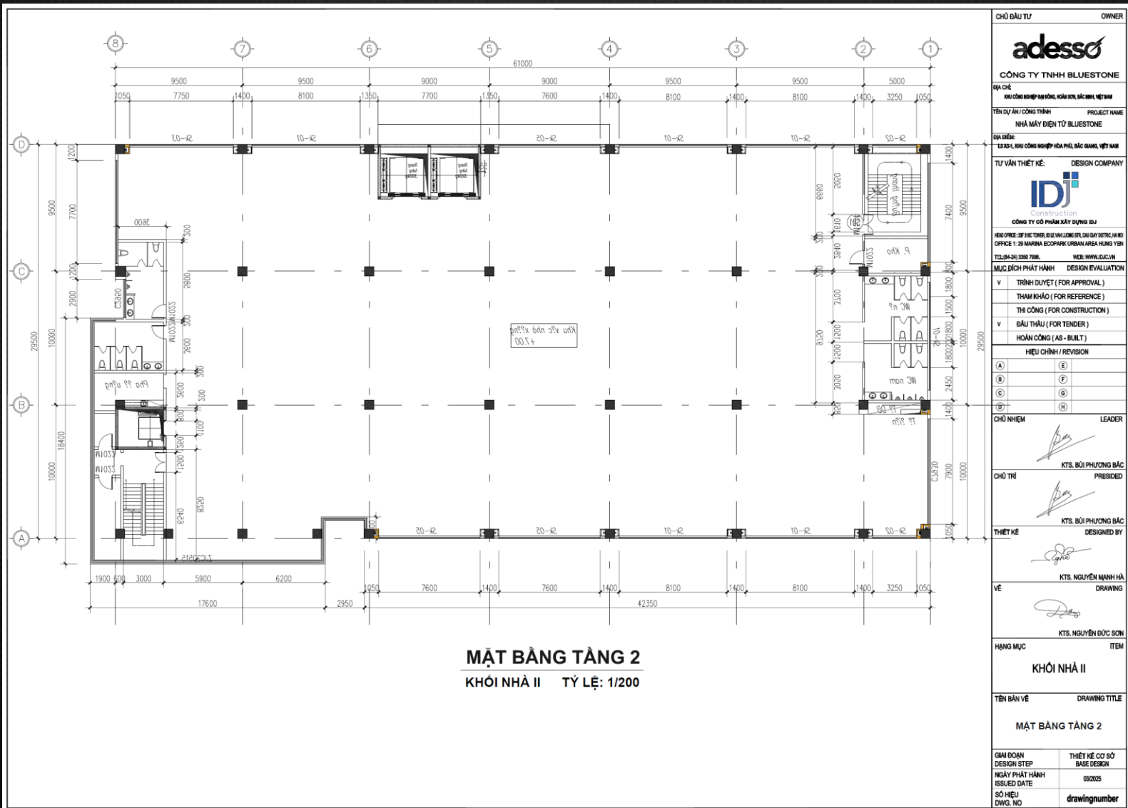
2号厂房2-5楼平面图 (建筑面积: 1860平方米/层)
