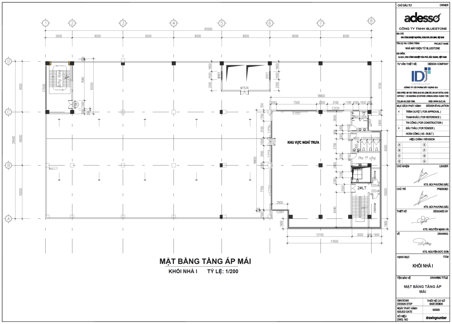
1号厂房6楼办公楼平面图 (建筑面积: 440平方米)
