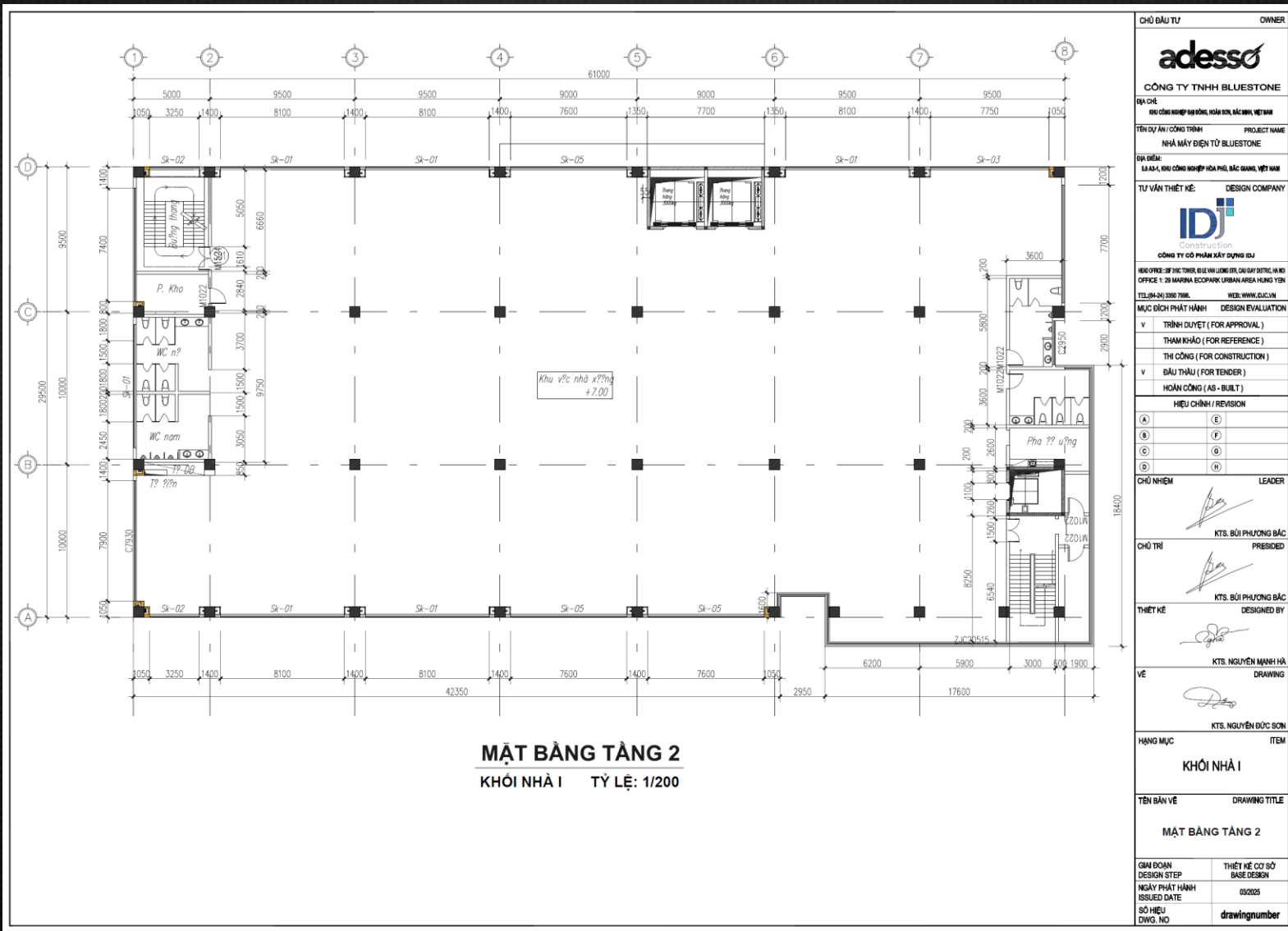
1号厂房2-5楼平面图 (建筑面积: 1860平方米/层)
